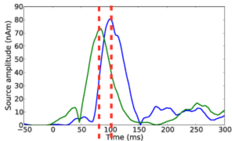
(d) \mathbf{X}_{\text{TF-MxNE}}^*
